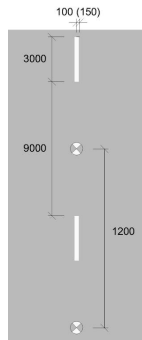
12 metre Module RRM 002A
