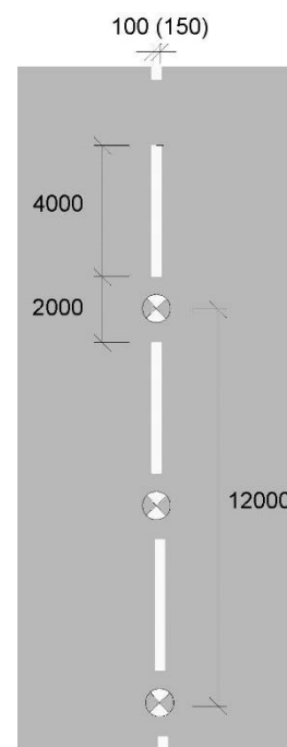
6 metre Module RRM 002C
