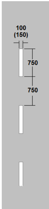
RRM 023 Broken Edge Line
