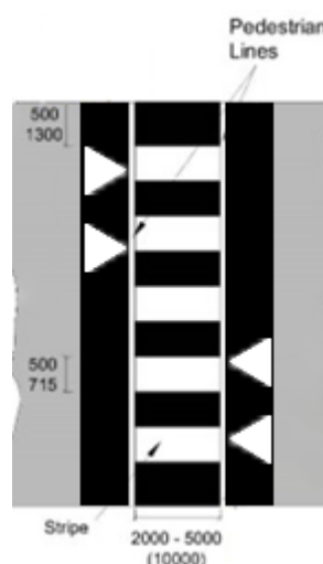
RPC 001A: Zebra Crossing (without beacons or RUS 066)
