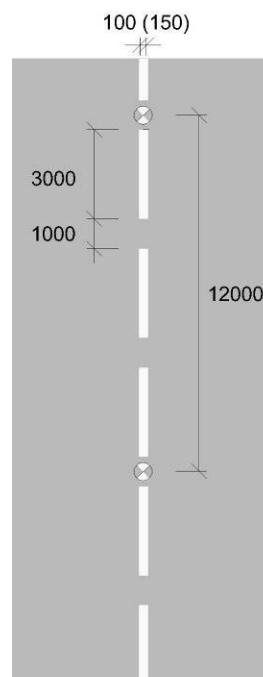
4 metre Module RRM 002D
