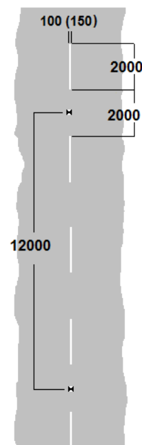
4 metre Module RRM 003B
