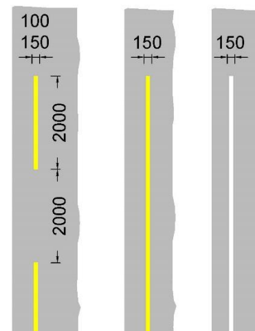
RRM 025 RRM 026 RRM 027
